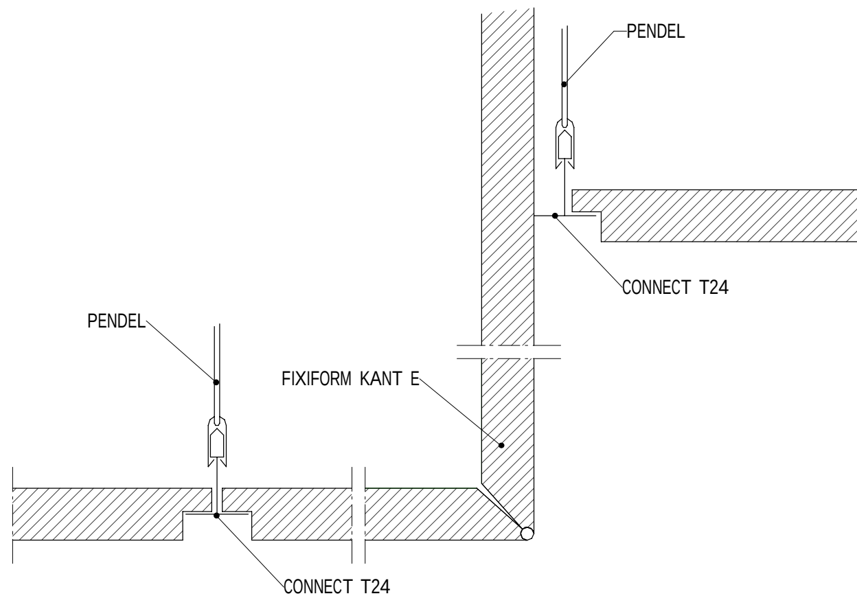
UTD05 - NIVÅSKILLNAD 1 : 2
