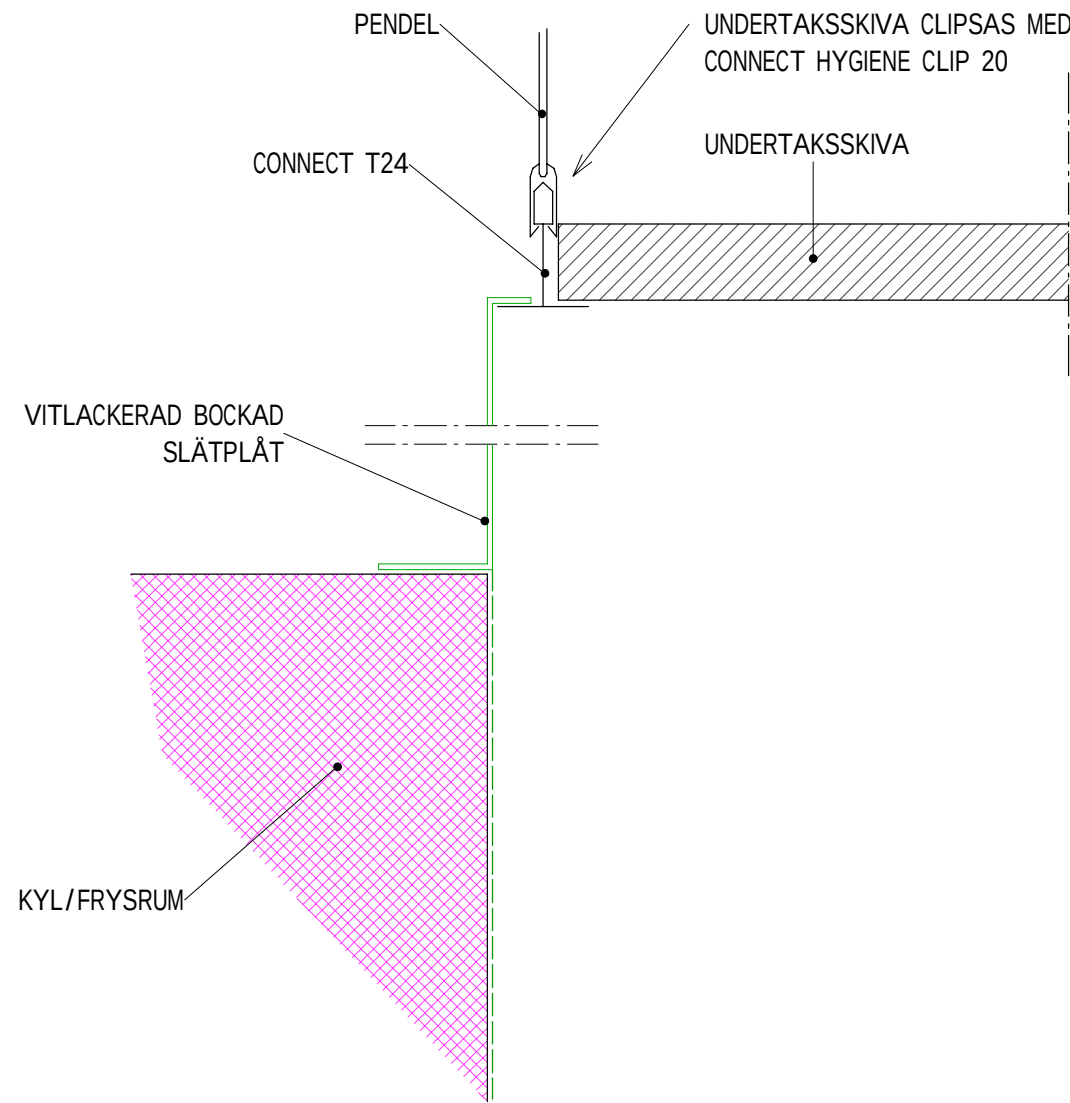
UTD02 - PRINCIPDETALJ ANSLUTNING MOT KYL-/FRYSRUM 1 : 2
