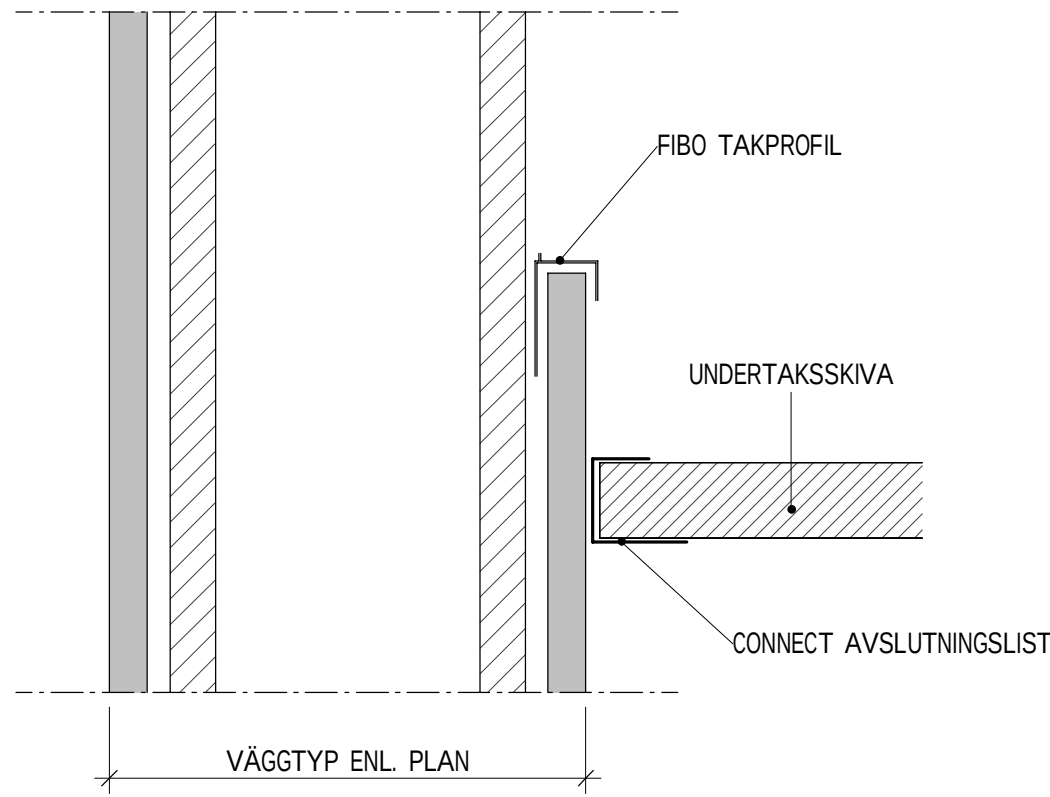
UTD01 - PRINCIPDETALJ ANSLUTNING MOT SPACE-PANEL 1 : 2
